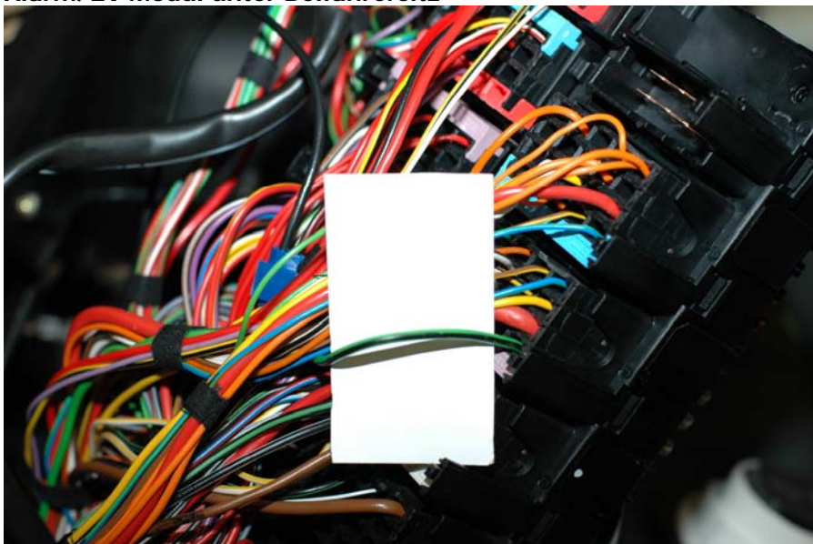
Sicherungskasten Sicherung 26 Treibstoffpumpe Stecker C Kammer 4 PIN 5 Rosa-Kennung
