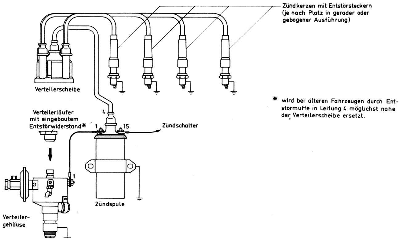
Prinzip-Schema einer UKW-Entstörung im Kraftfahrzeug
