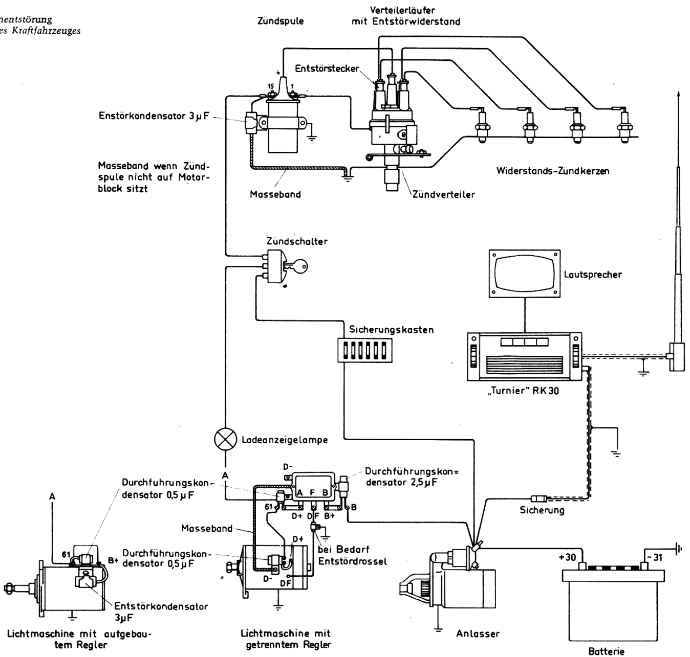
Prinzip-Schema einer UKW-Entstörung im Kraftfahrzeug
