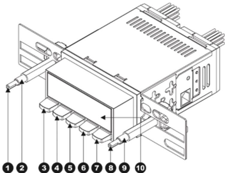
Abbildung 9 - Bedienelement
