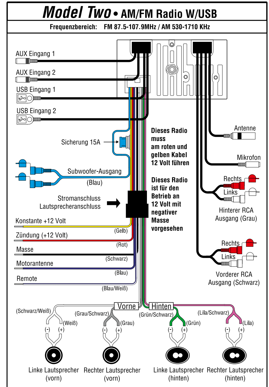
Abbildung 8 - Kabelplan
