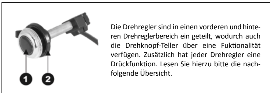
Abbildung 10 - Drehregler mit Drehknöpfen
